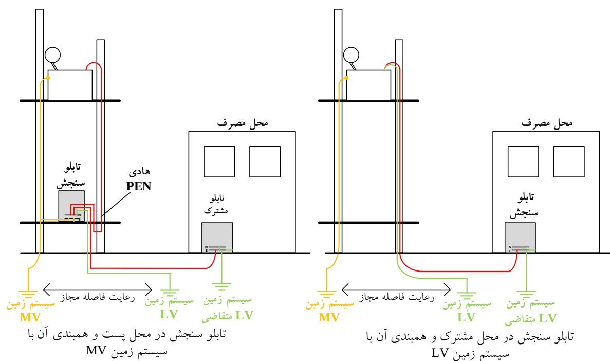
شکل ۴-۲۱- طرحواره اتصال زمین در تغذیه هوایی مشترکین
