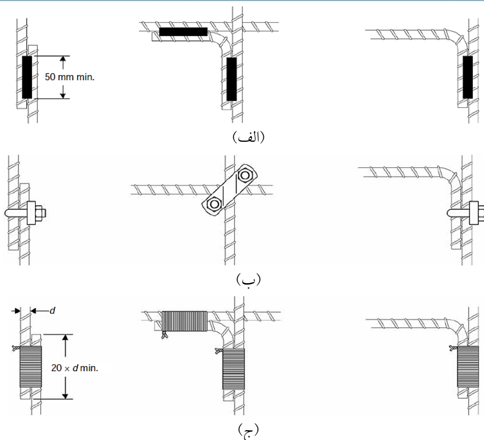
شکل ۴-۱۵- اتصالات مورد تایید استاندارد IEC62305-3 برای اتصال میلگرد همبندی و میلگردهای سازه، (الف): اتصال با استفاده از جوشکاری، (ب): اتصال با استفاده از کلمپ و (ج): اتصال با استفاده از سیم بندی
