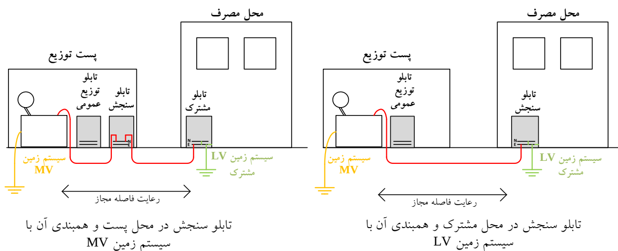
شکل ۴-۲۲- طرحواره اتصال زمین در تغذیه زمینی مشترکین
